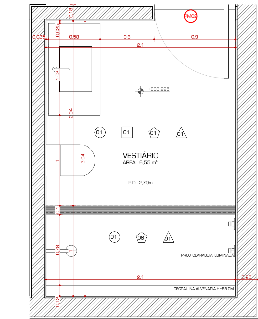
PLANTA AMPLIADA VESTIÁRIO
