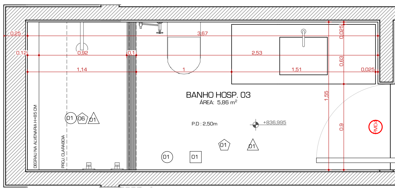
PLANTA AMPLIADA BANHO HOSP. 03
