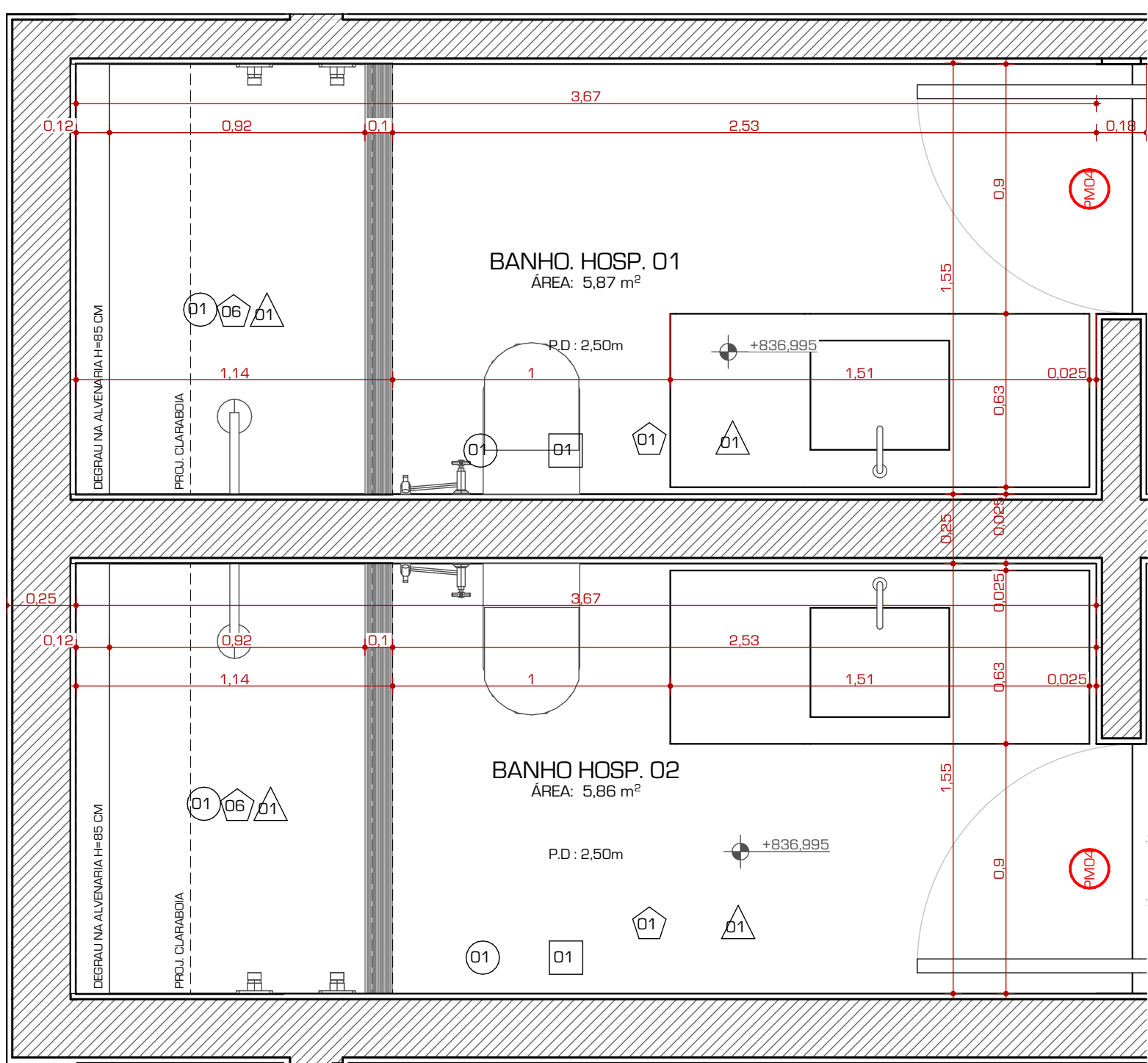
PLANTA AMPLIADA BANHO HOSP. 01 E 02
