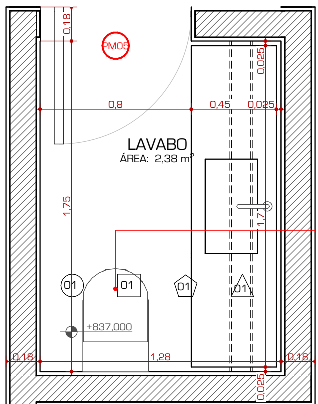
PLANTA AMPLIADA LAVABO
