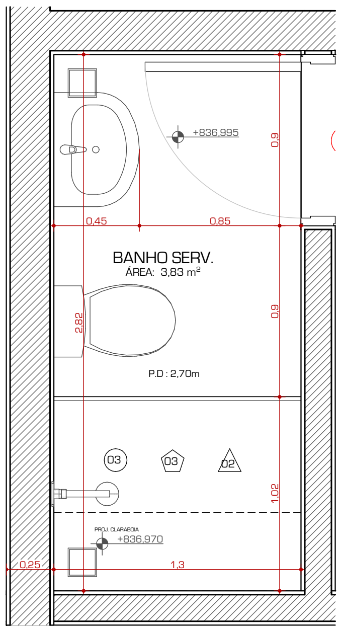
PLANTA AMPLIADA BANHO SERVIÇO
